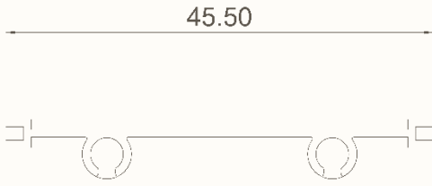
Alüminyum Led Sürgü (72 WATT)
